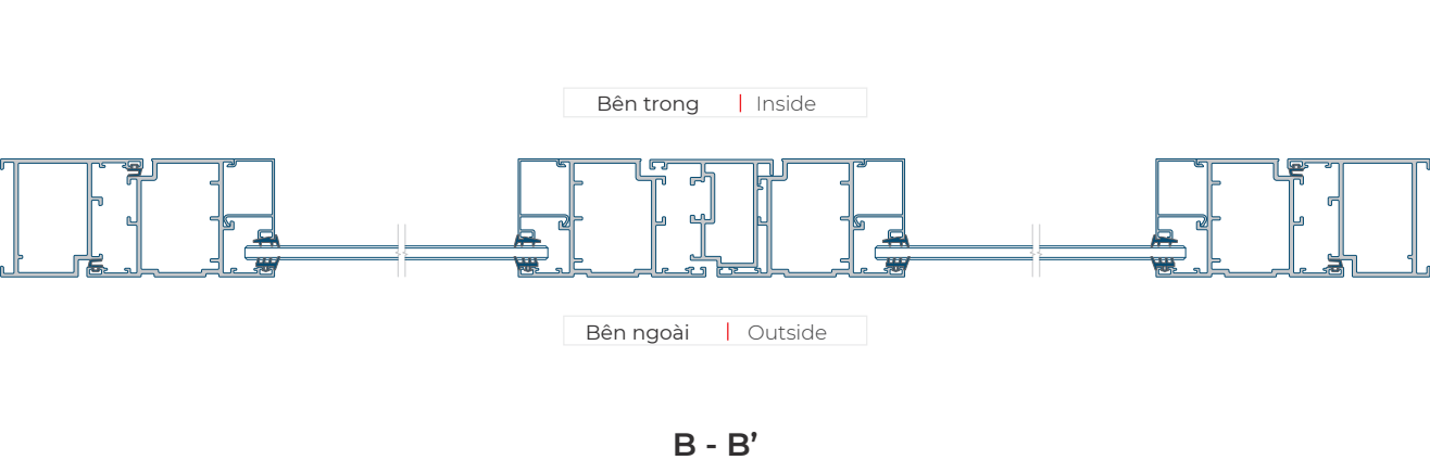
Mặt cắt ngang | Horizontal section
