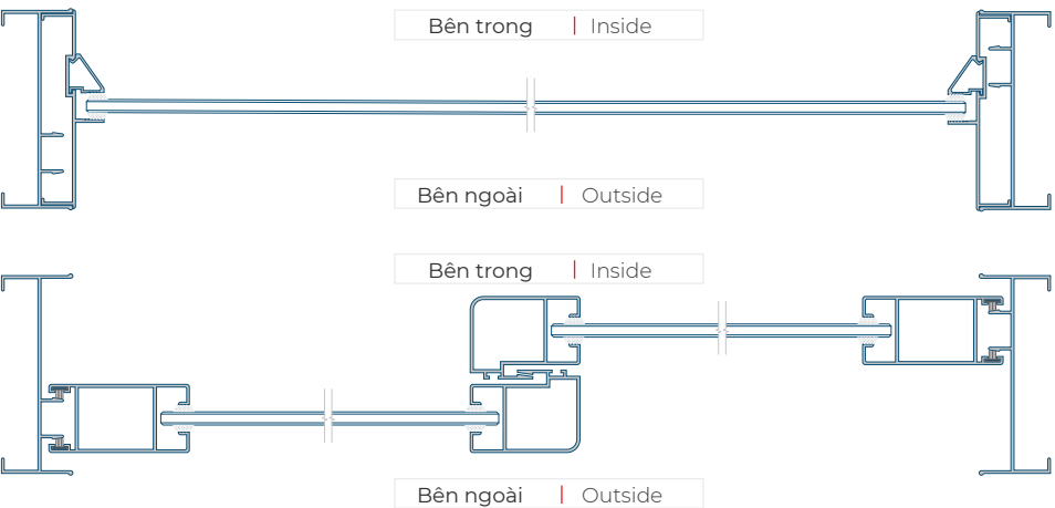
Mặt cắt ngang | Horizontal section
