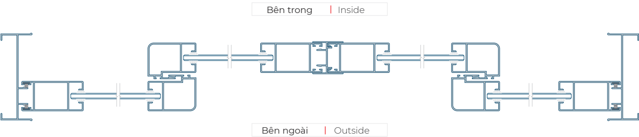
B - B'
