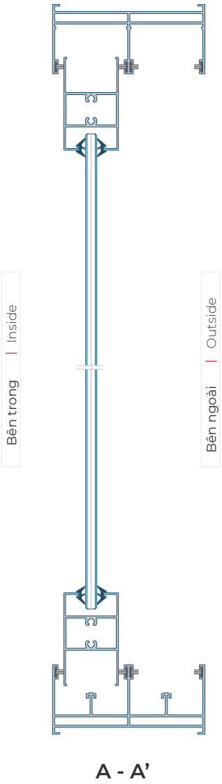
Mặt cắt dọc | Vertical Section
