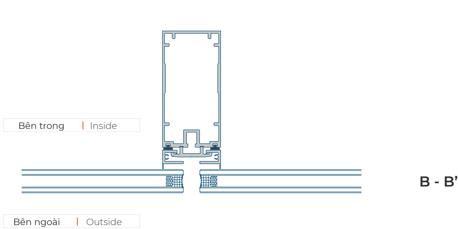
Mặt cắt ngang | Horizontal section
