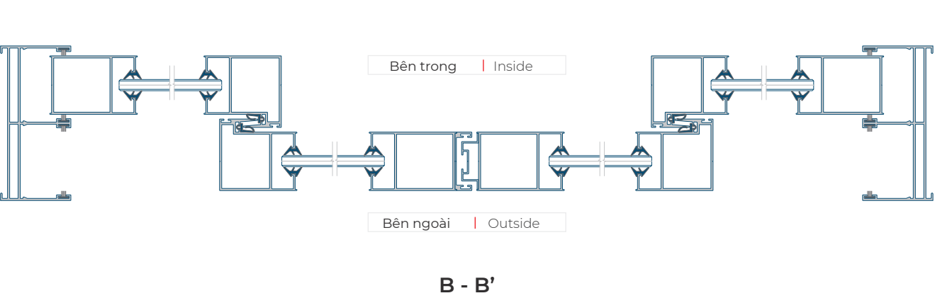
Mặt cắt ngang | Horizontal section
