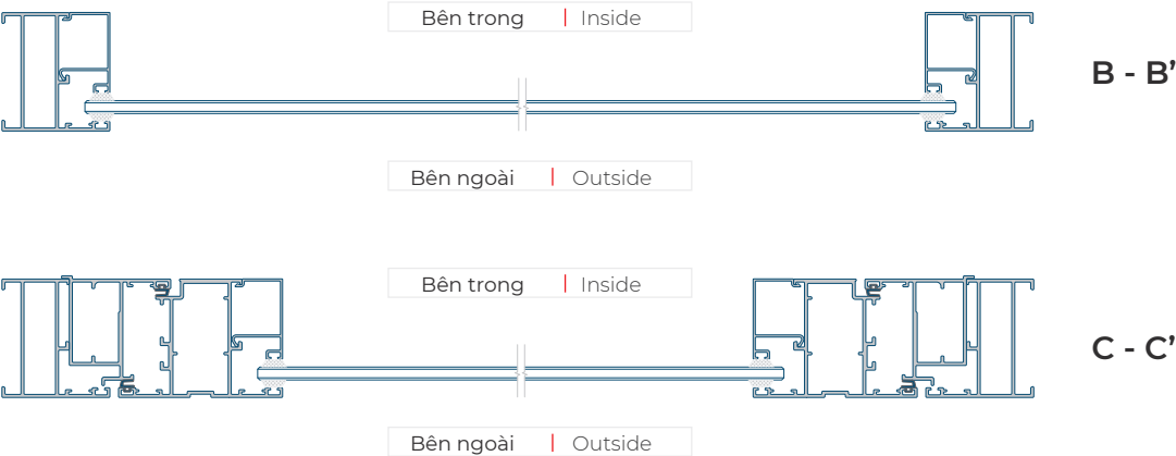
Mặt cắt ngang | Horizontal section
